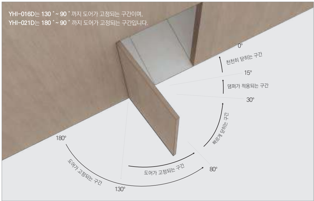
YHI-021 / YHI-021D (1P) [실버] 히든 경첩 (일반형 / 댄퍼형)
