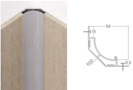
30 인코너 라운드 64 x 64 x 2,400 (mm)
