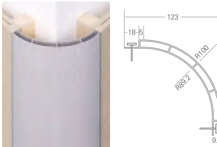
100 아웃코너 라운드 * 인코너 활용 가능 123 x 123 x 2,400 (mm)
