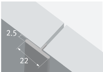
AL 양개형 바람막이 몰딩 적용 가능 색상: 전 색상 시트 래핑
