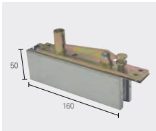
글래스 피봇힌지(댁퍼형) 상부
