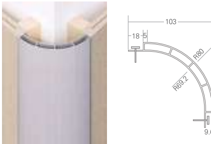
80 아웃코너 라운드 * 인코너 활용 가능 103 x 103 x 2,400 (mm)
