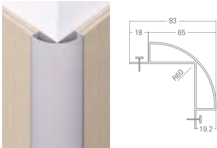
60 아웃코너 라운드 83 x 83 x 2,400 (mm)
