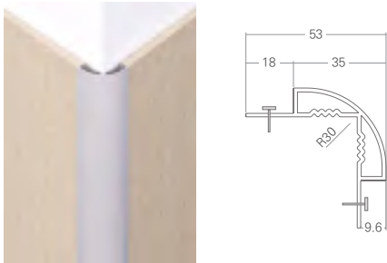
30 아웃코너 라운드 53 x 53 x 2,400 (mm)
